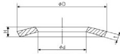
碟形弹簧的形状·尺寸
